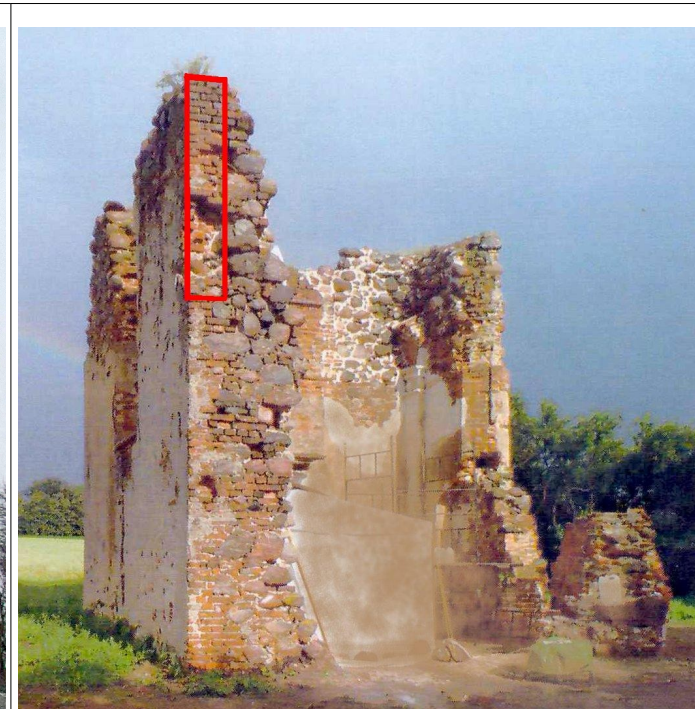
Ilustracja 3: Ściana zachodnia
